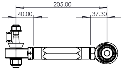
MIN LENGTH - 205MM
